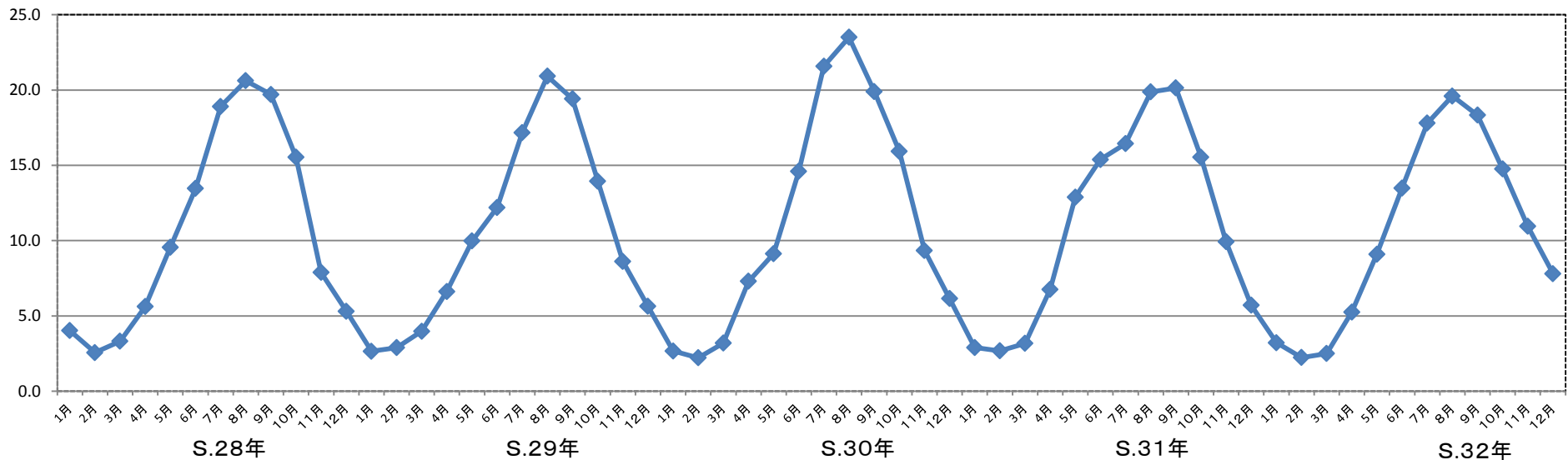
昭和28年～32年平均水温
