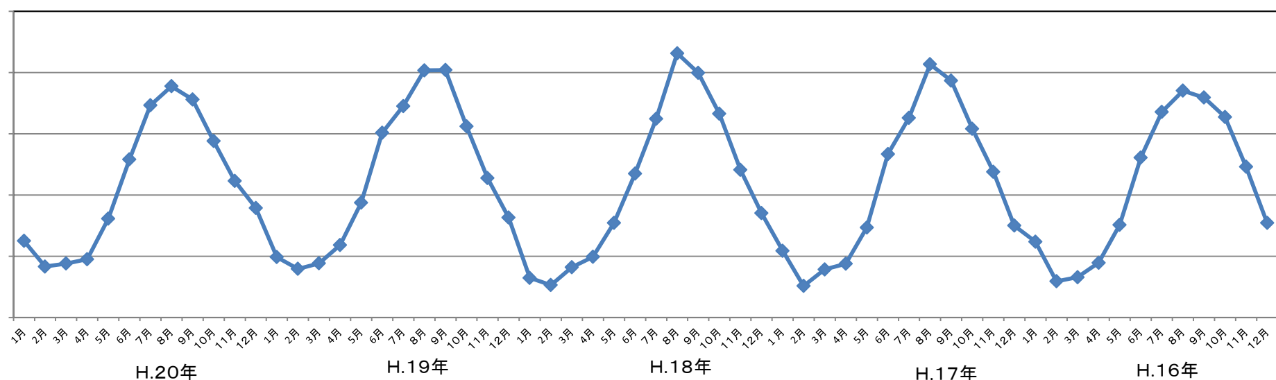
平成20年～16年平均水温
