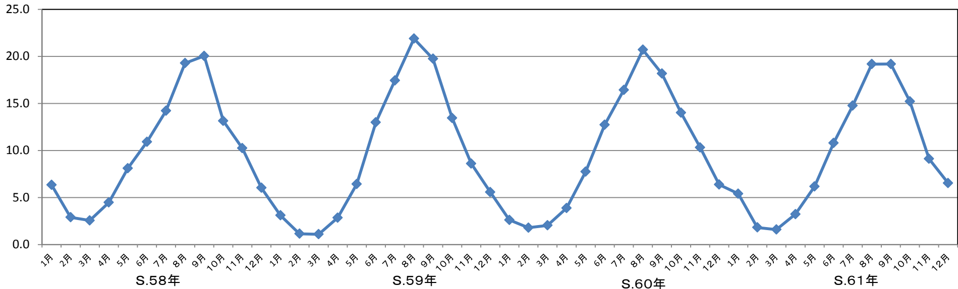
昭和58年～61年水温平均
