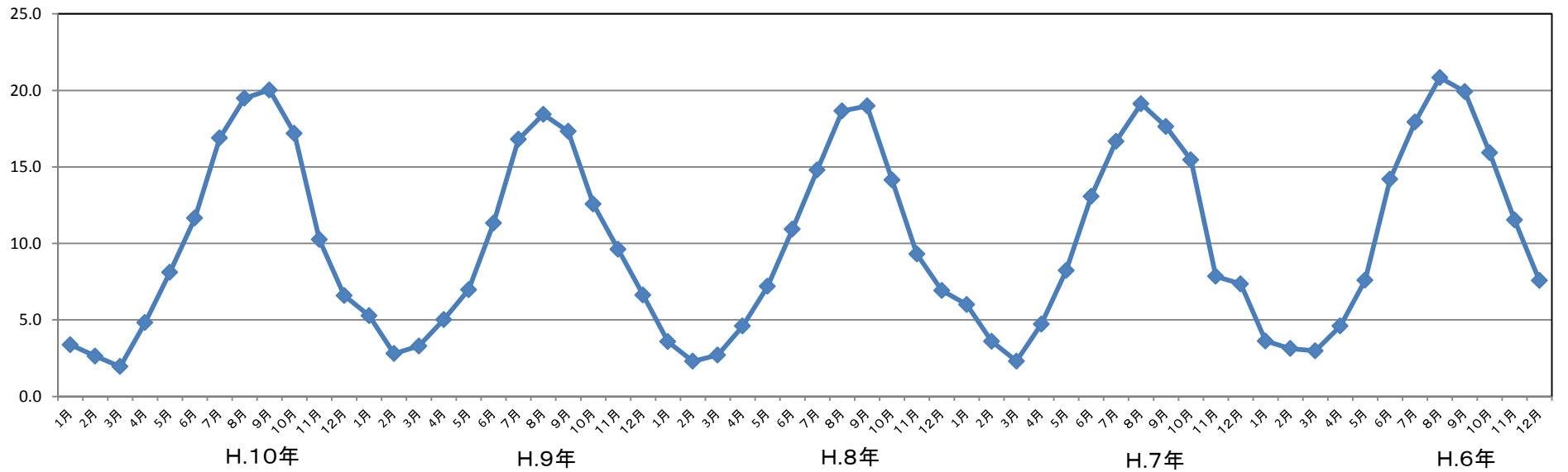
平成10年～6年平均水温
