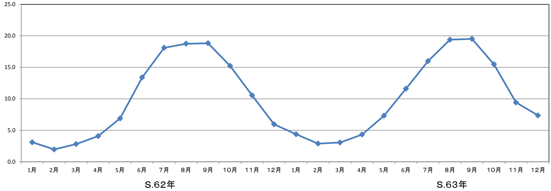
昭和62年～63年水温平均
