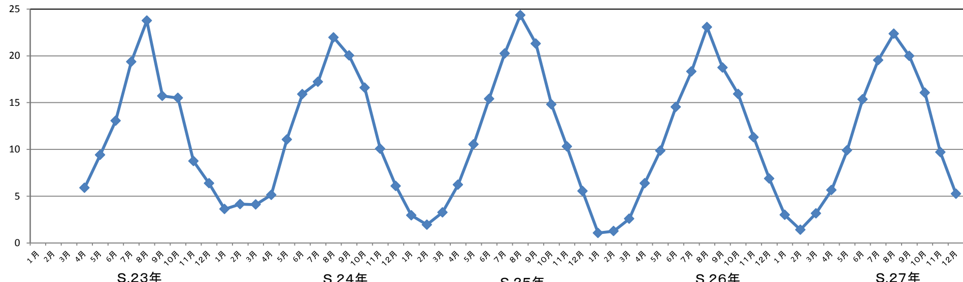
昭和23年～27年水温平均
