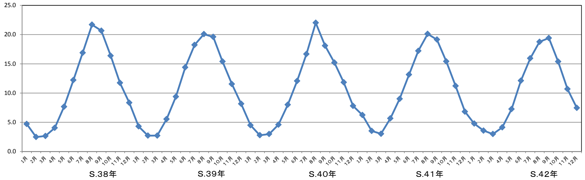
昭和38年～42年水温平均
