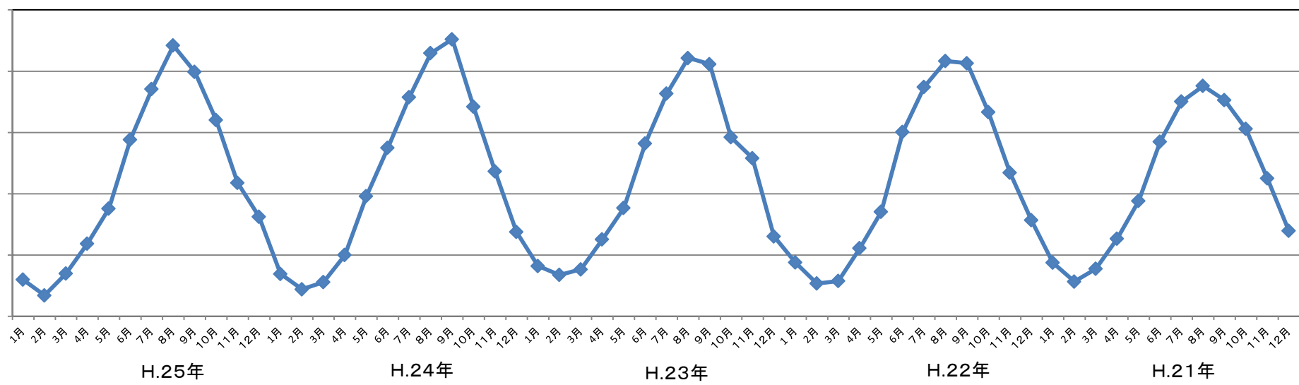
平成25年～21年平均水温
