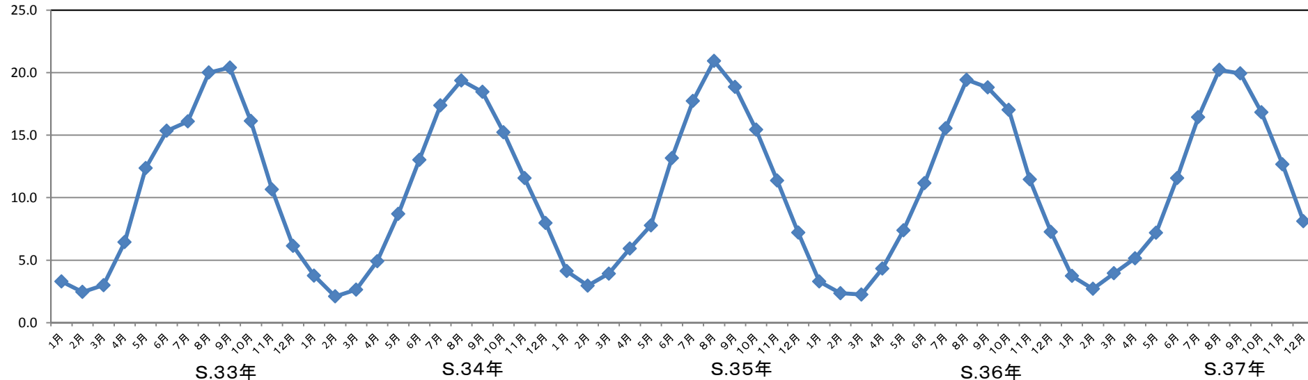
昭和33年～37年水温平均
