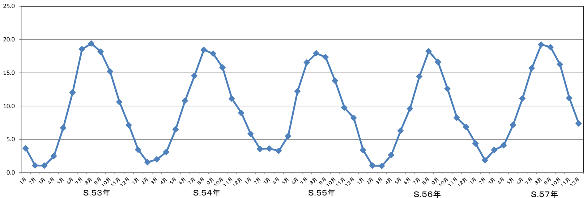
昭和53年～57年水温平均
