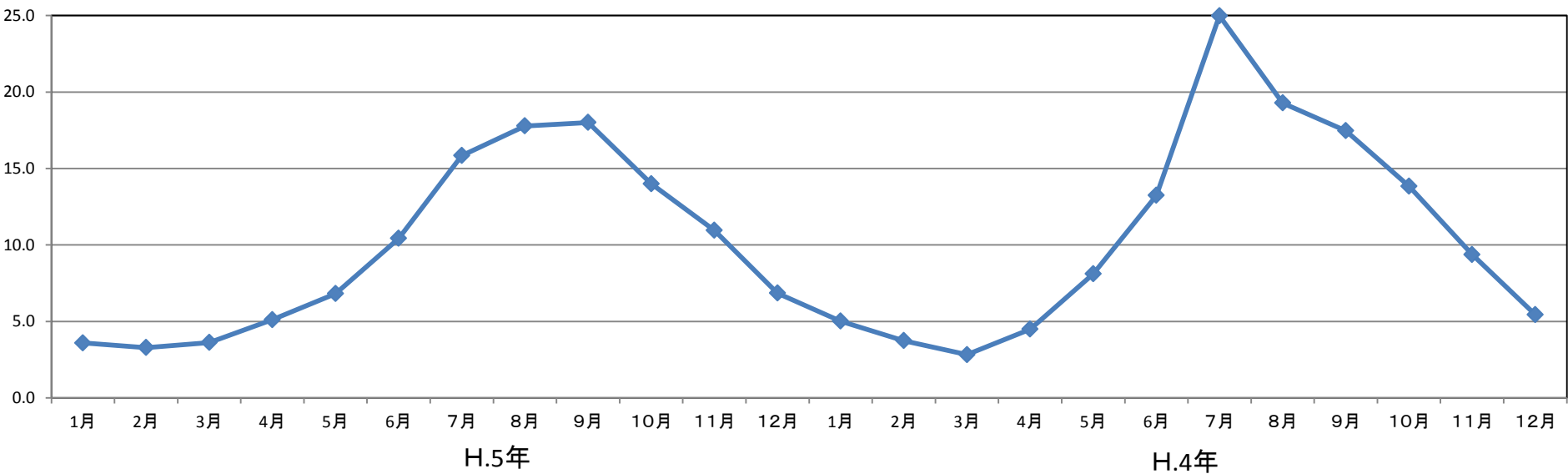
平成5年～4年水温平均
