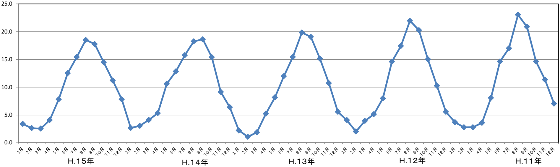
平成15年～11年平均水温
